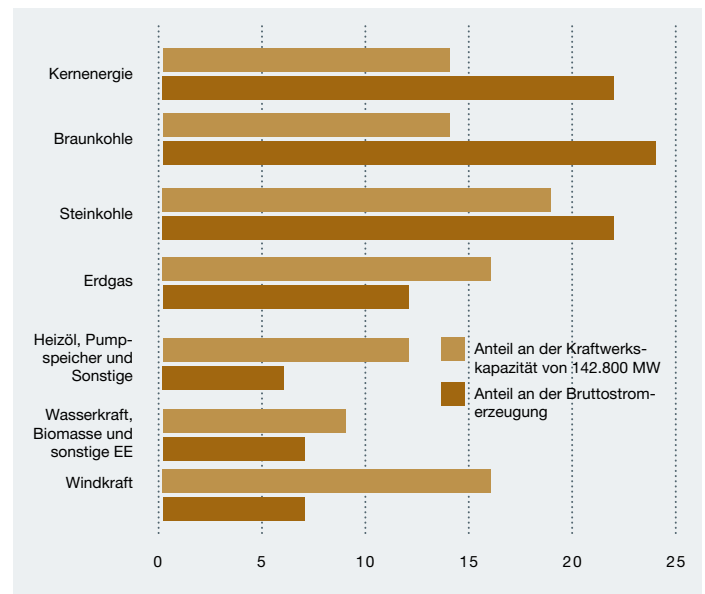
Anteile der Energieträger an Kraftwerkskapazität und Bruttostromerzeugung 2007 (in %)
